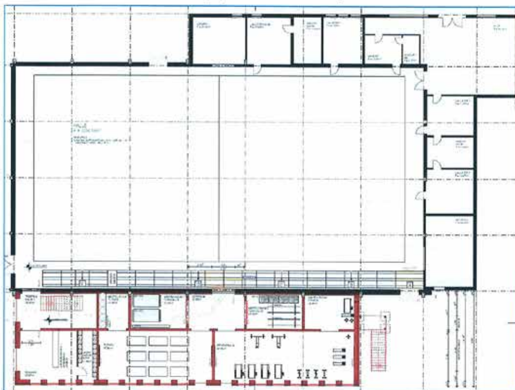
Abb. 8: Grundriss Entwurfszeichnung Sporthallenerweiterung
